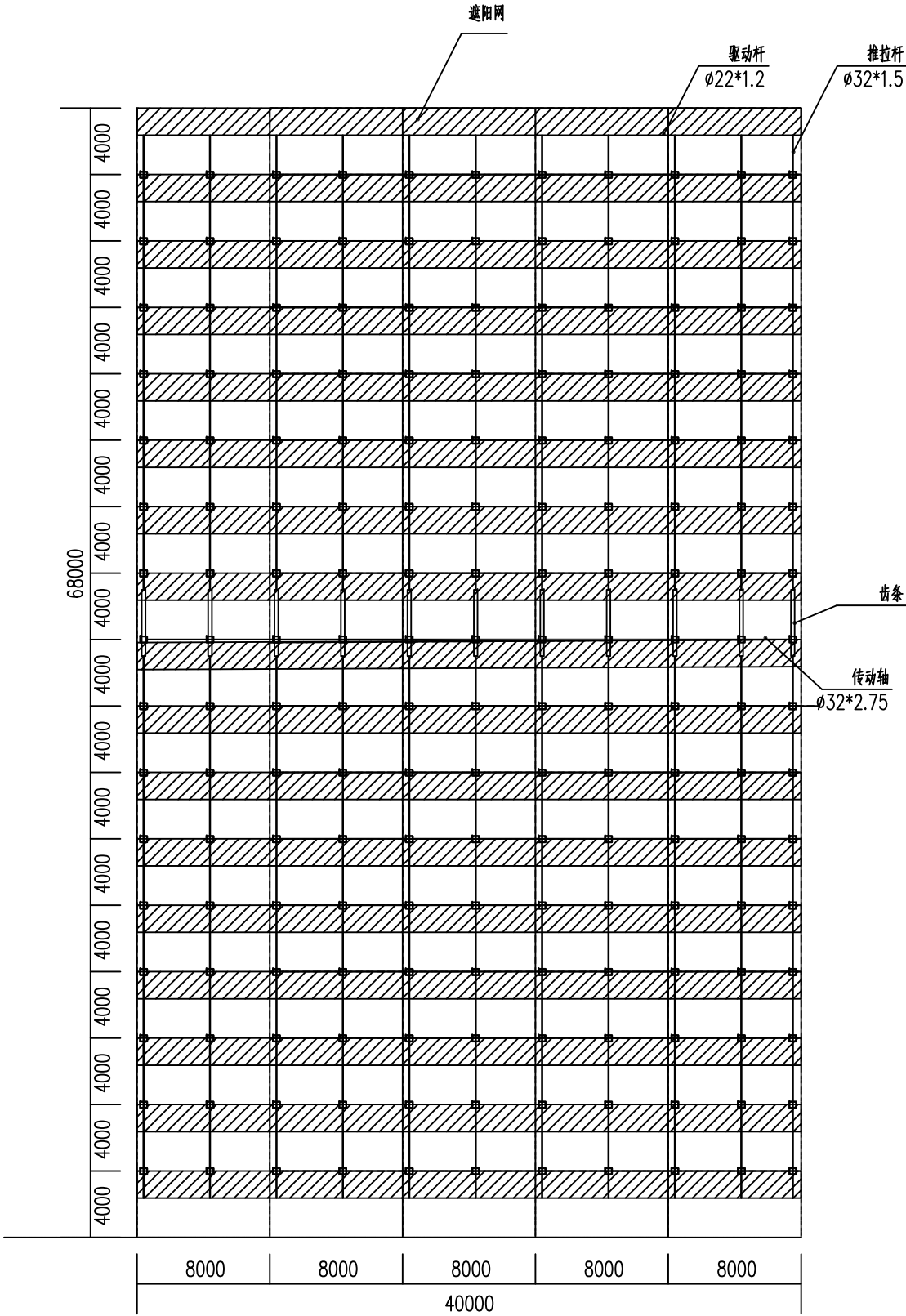
3#外遮阳系统平面布置图
