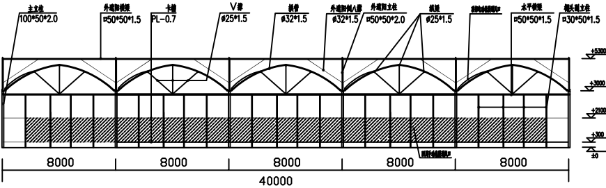
2#端面正视图
