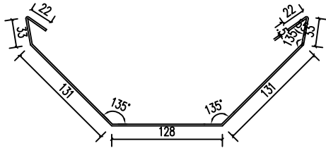
水槽大样图
