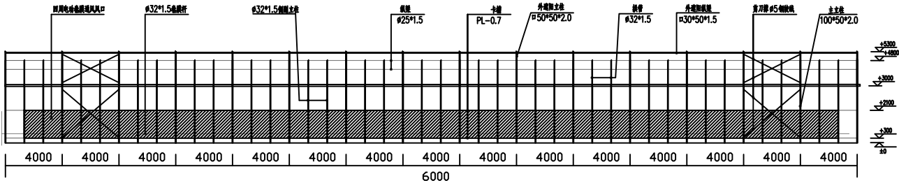
2#侧面正视图
