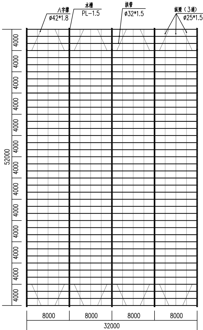
5#屋面钢架布置图
