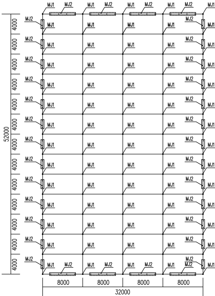
1#独立基础平面布置图
