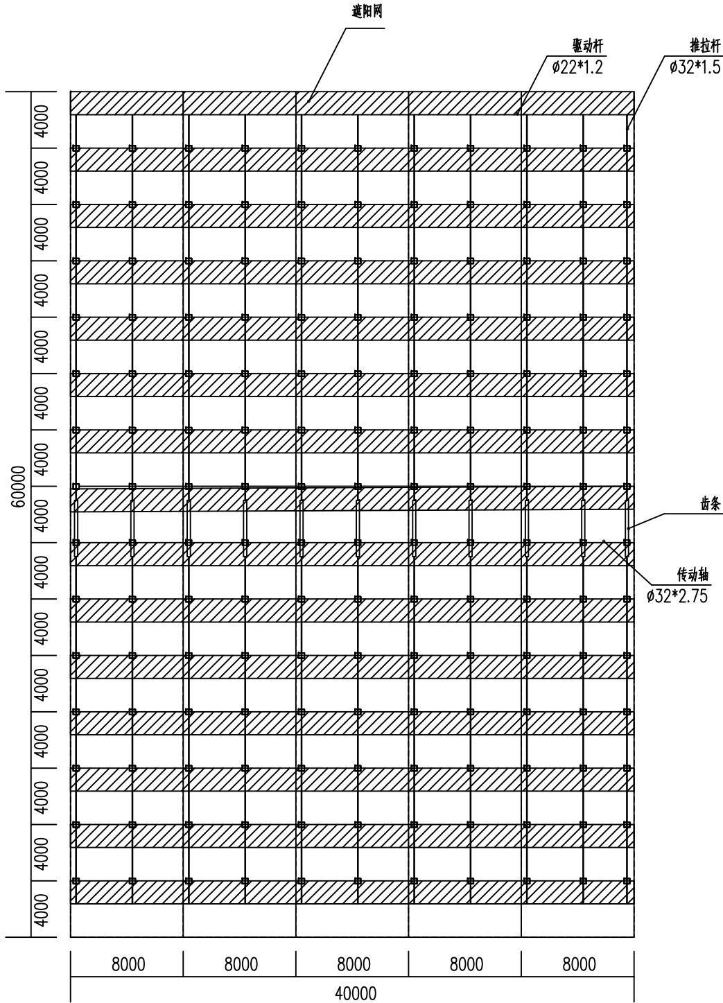
2#外遮阳系统平面布置图
