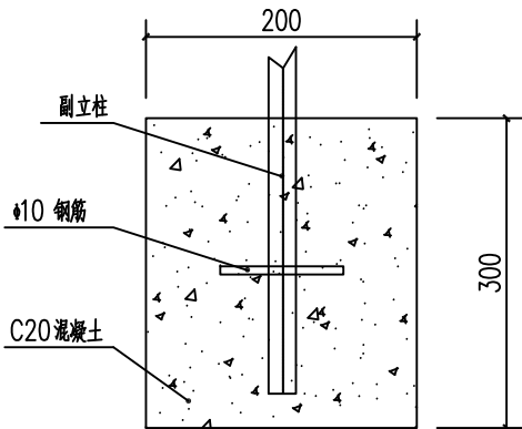
副立柱基础剖面图
