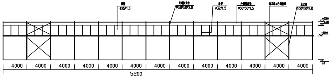
5#侧面剖视图
