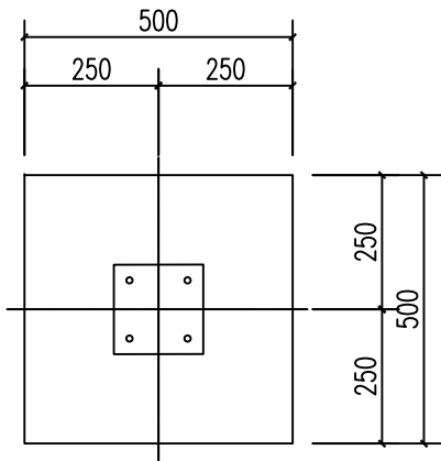
主立柱基础平面图
