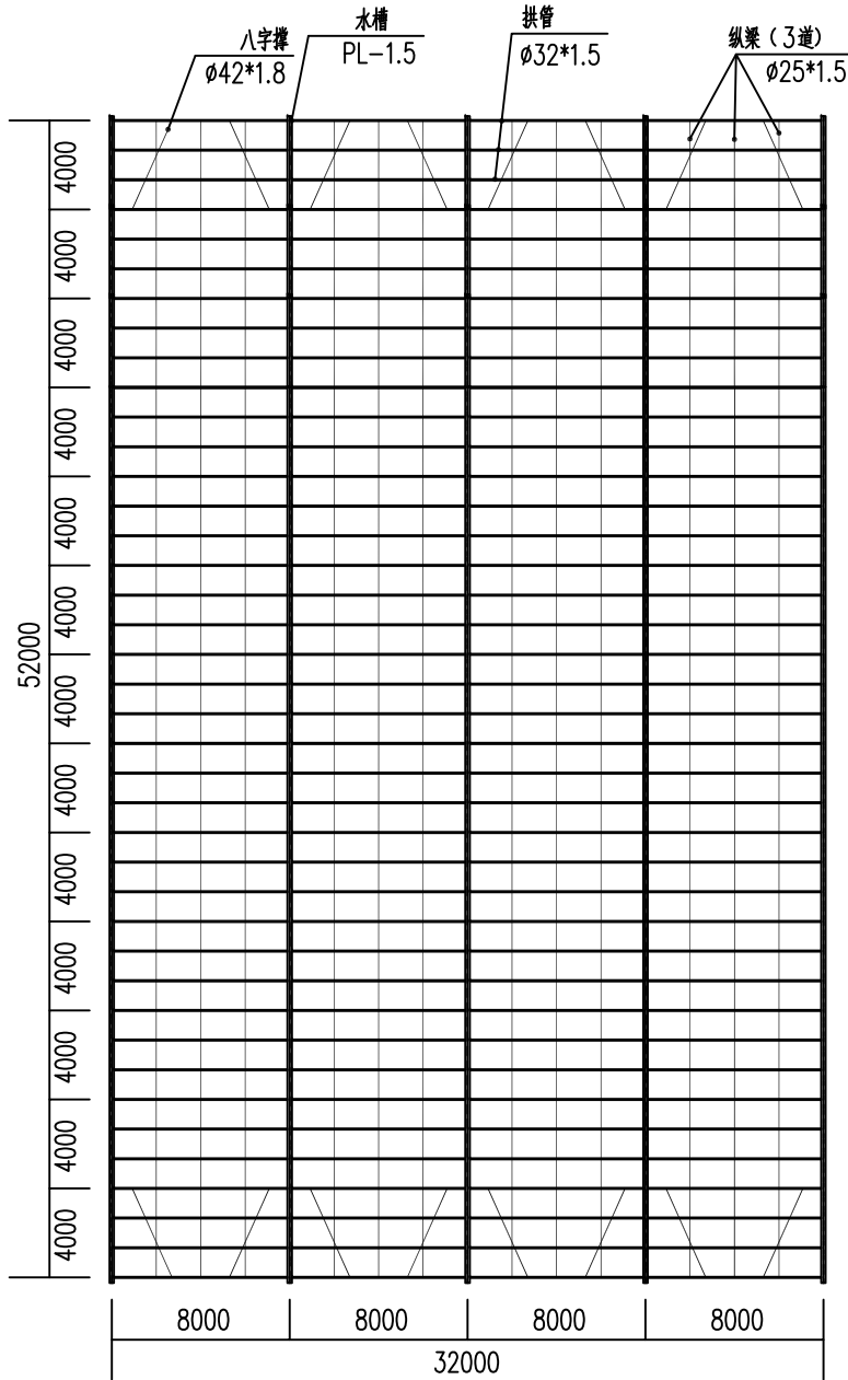
1#屋面钢架布置图
