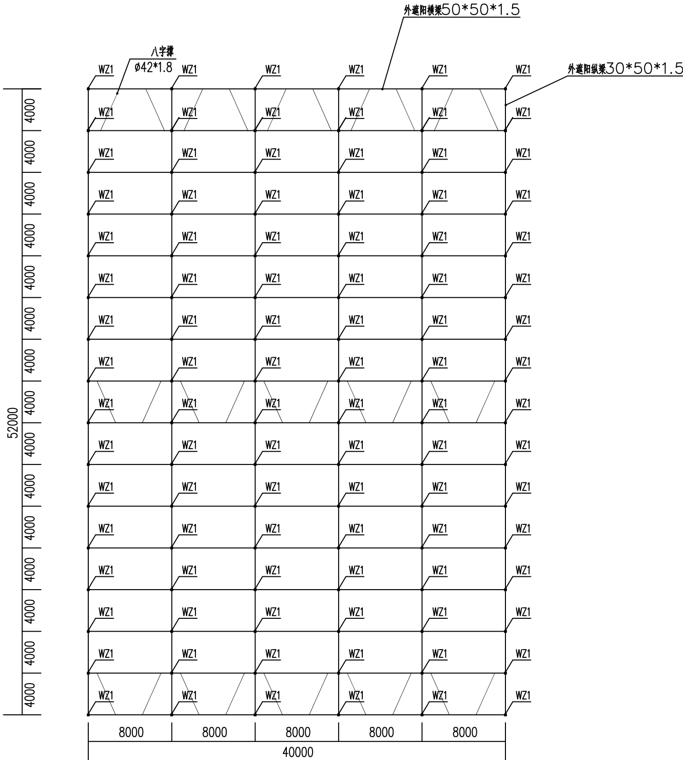
2#外遮阳钢架布置图
