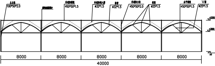
2#端面剖视图
