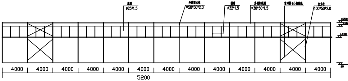
1#侧面剖视图
