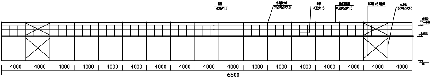
3#侧面剖视图
