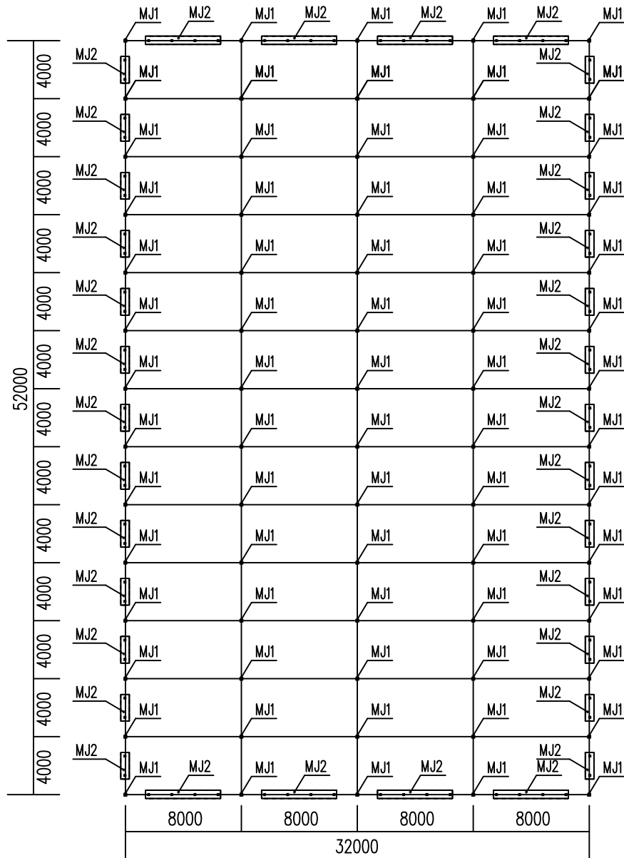
4#独立基础平面布置图
