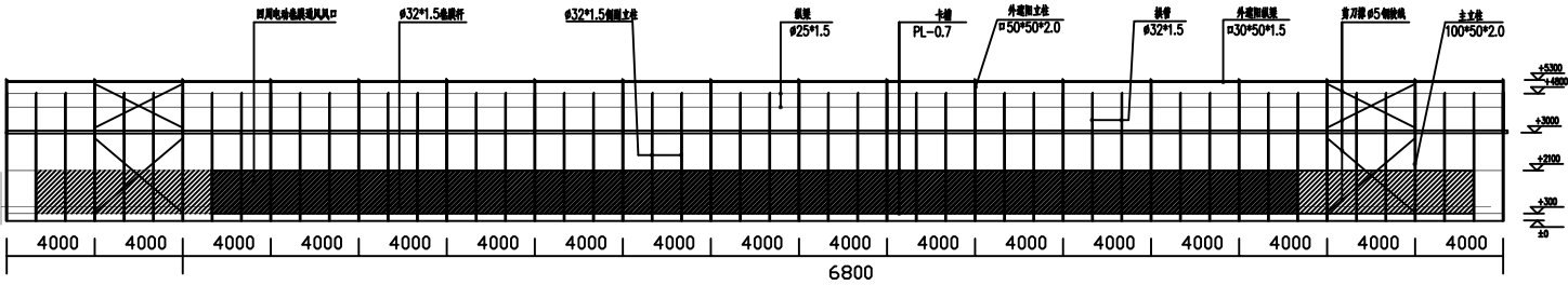
3#侧面正视图
