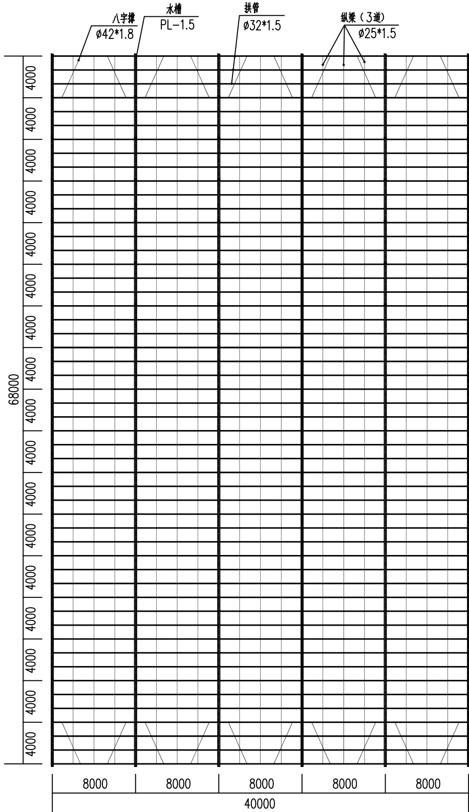
3#屋面钢架布置图
