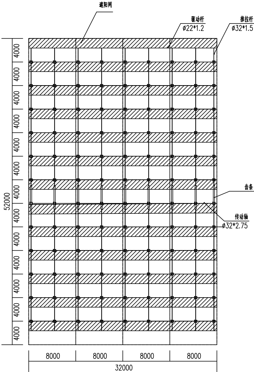
5#外遮阳系统平面布置图
