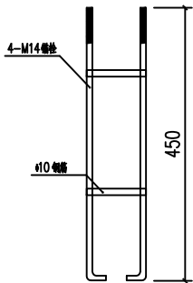
预埋锚栓剖面图
