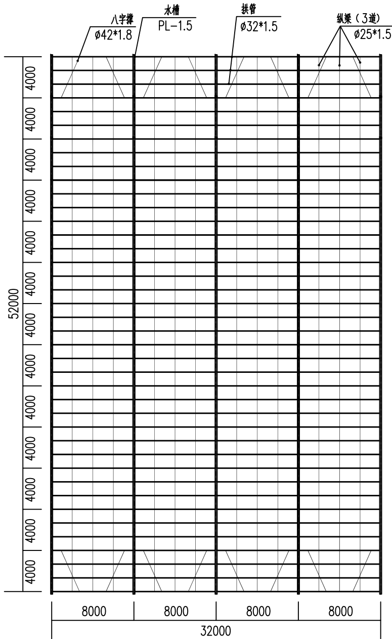
4#屋面钢架布置图
