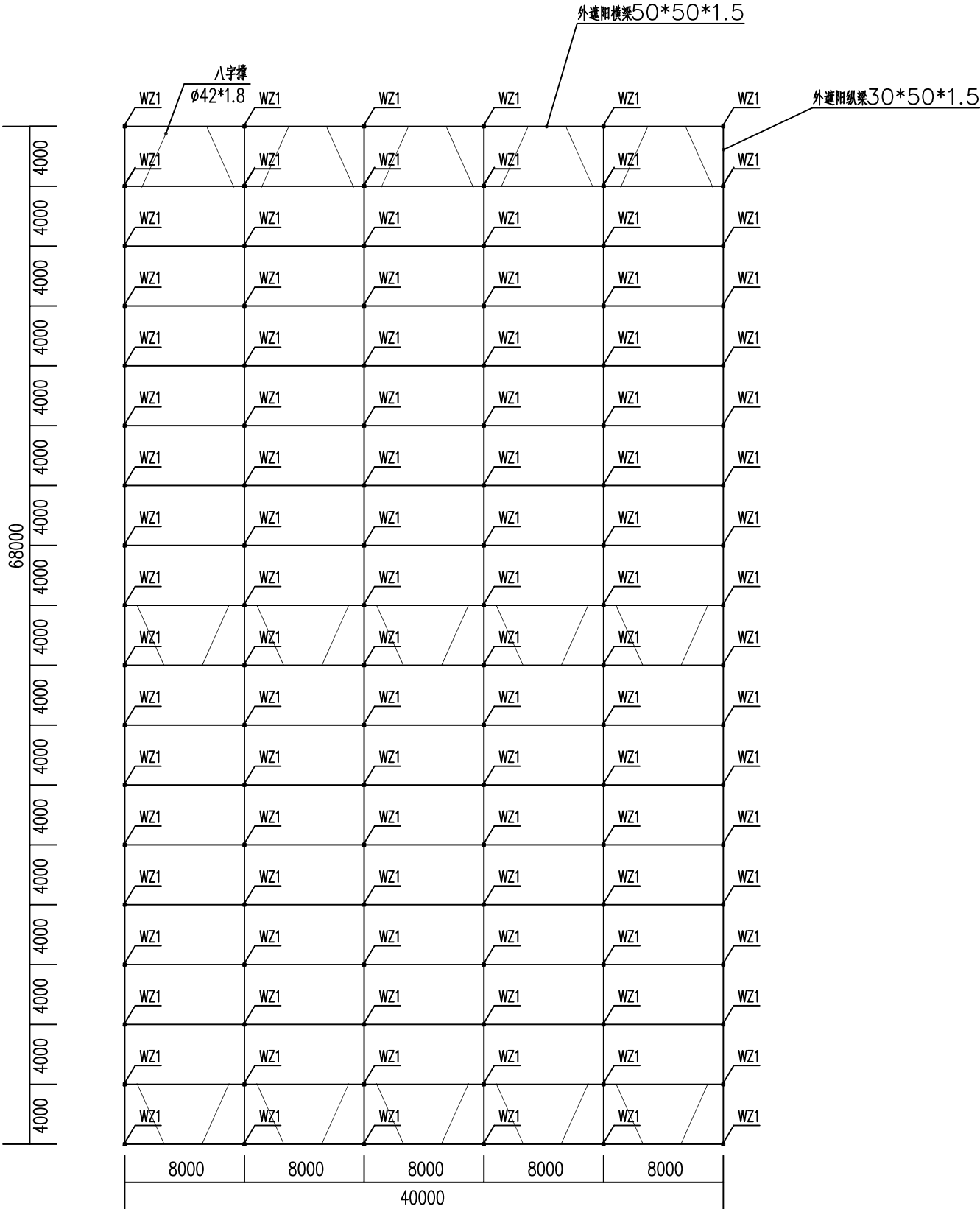
3#外遮阳钢架布置图
