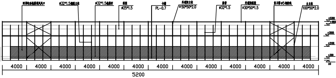
1#侧面正视图
