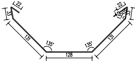
水槽大样图
