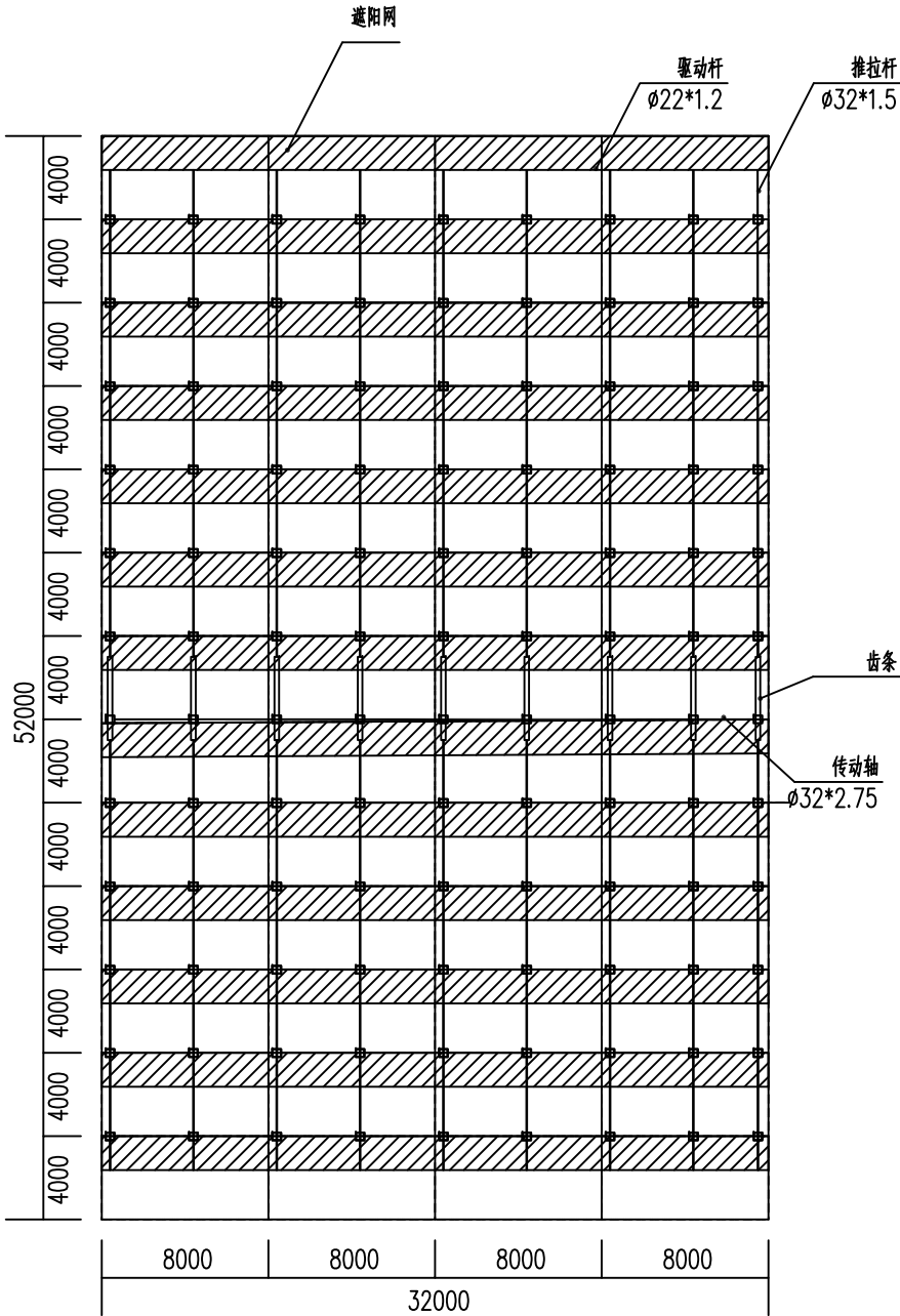
4#外遮阳系统平面布置图
