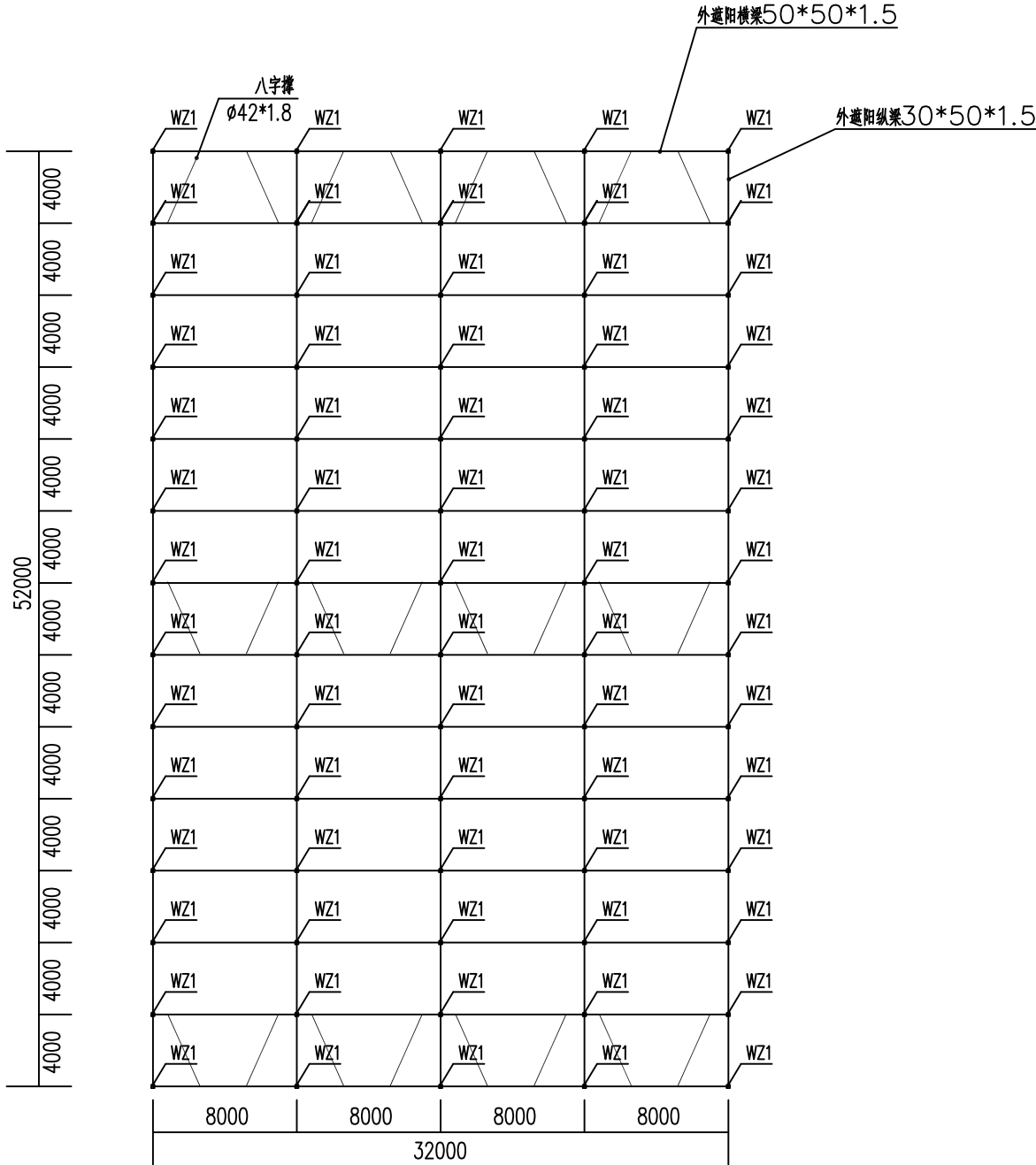
1#外遮阳钢架布置图
