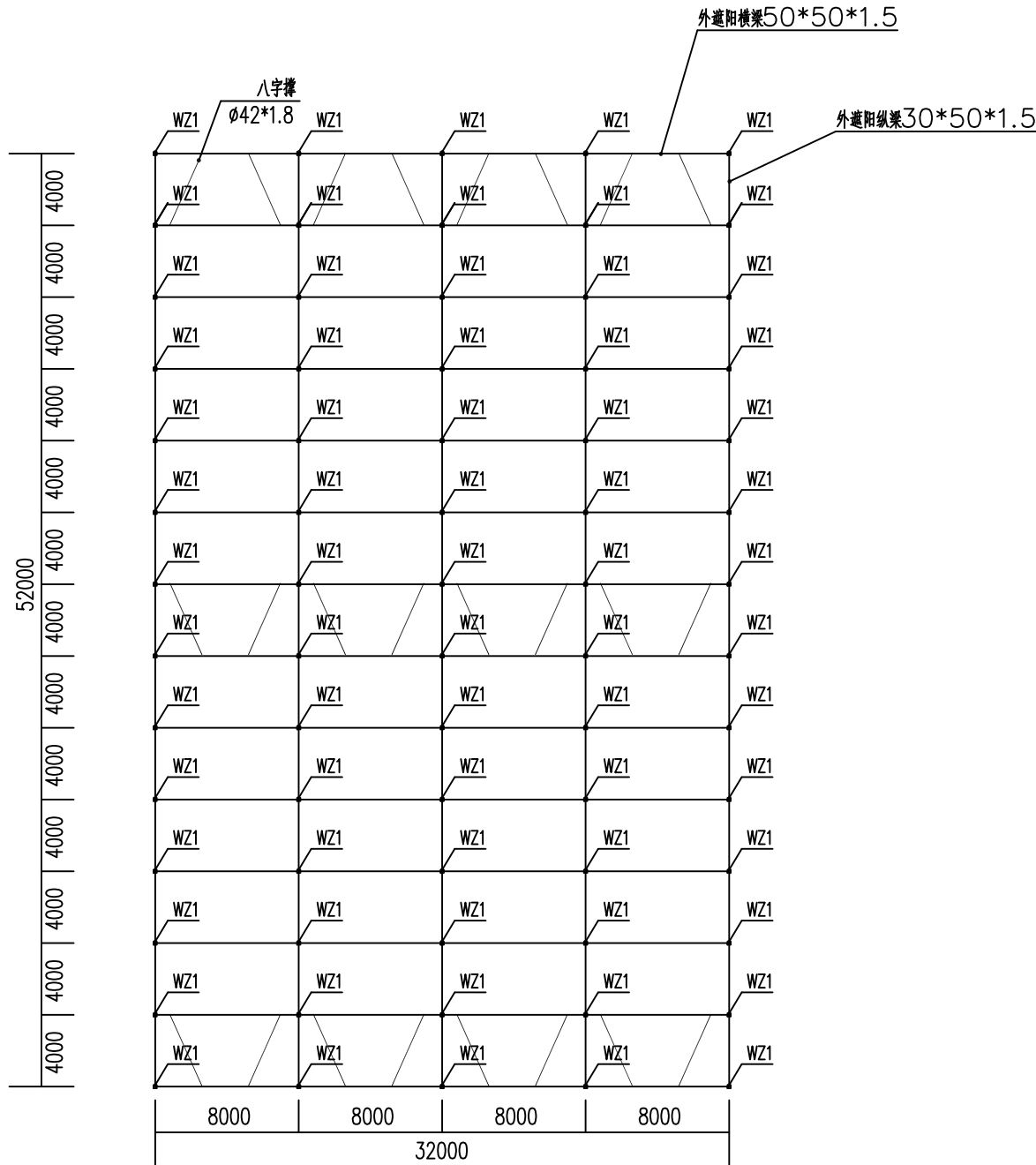
4#外遮阳钢架布置图
