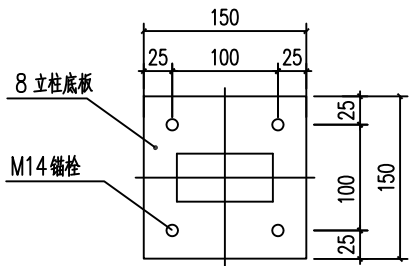
主立柱底座平面图
