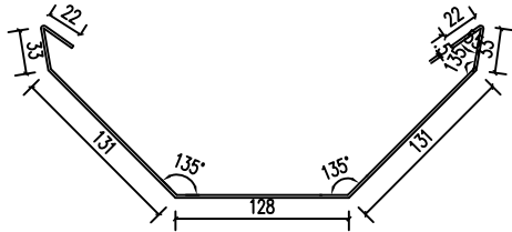
水槽大样图
