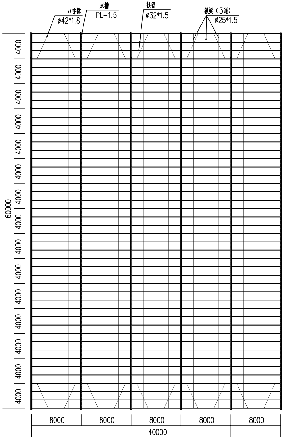
2#屋面钢架布置图
