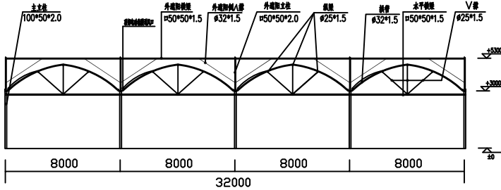
1#端面剖视图
