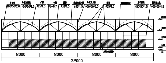
4#端面正视图
