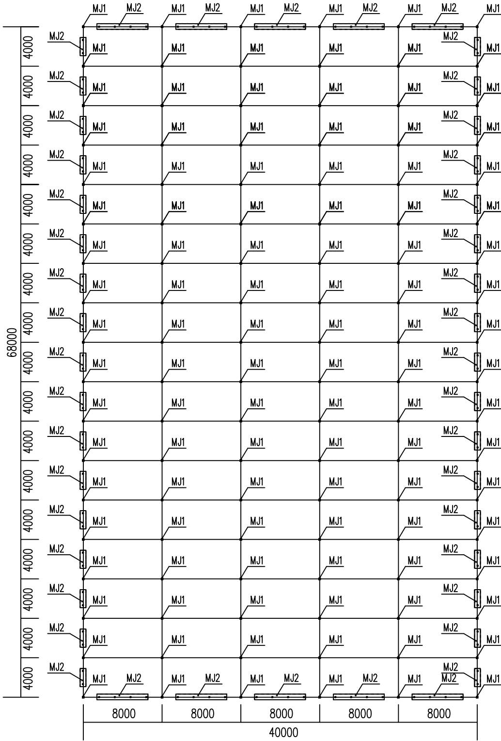
3#独立基础平面布置图
