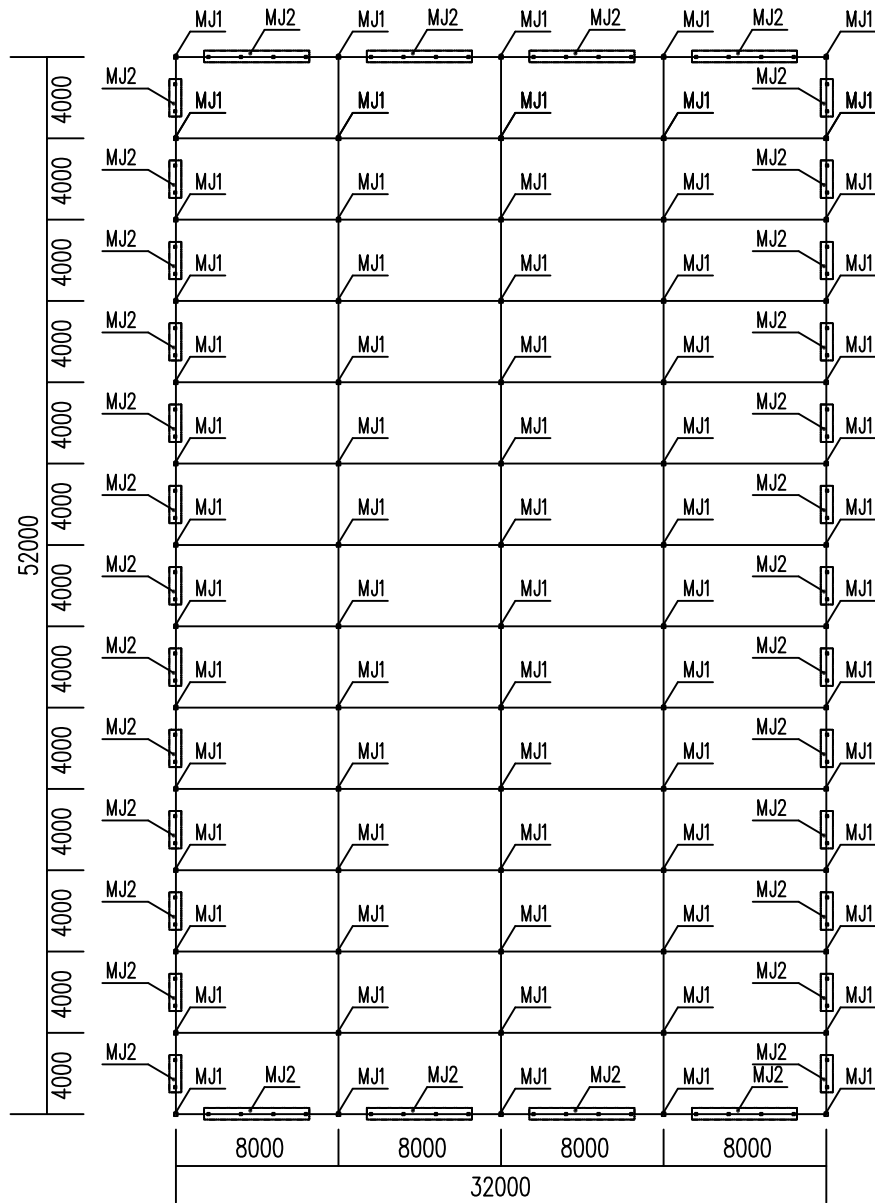
5#独立基础平面布置图
