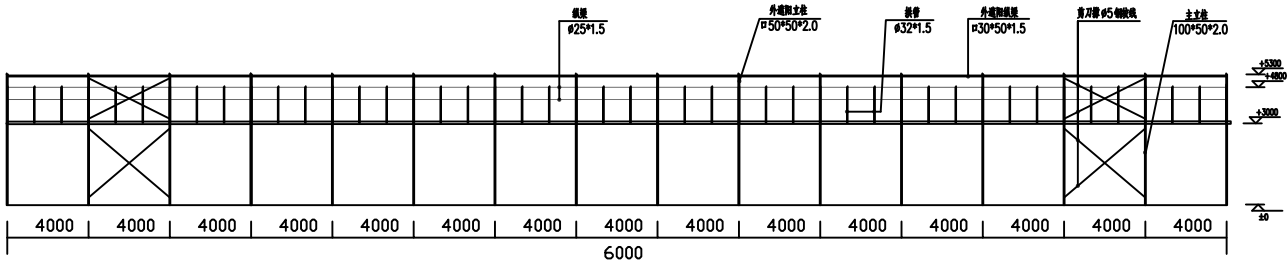
2#侧面剖视图
