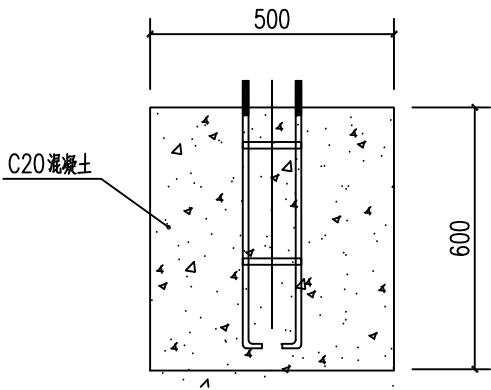
主立柱基础剖面图
